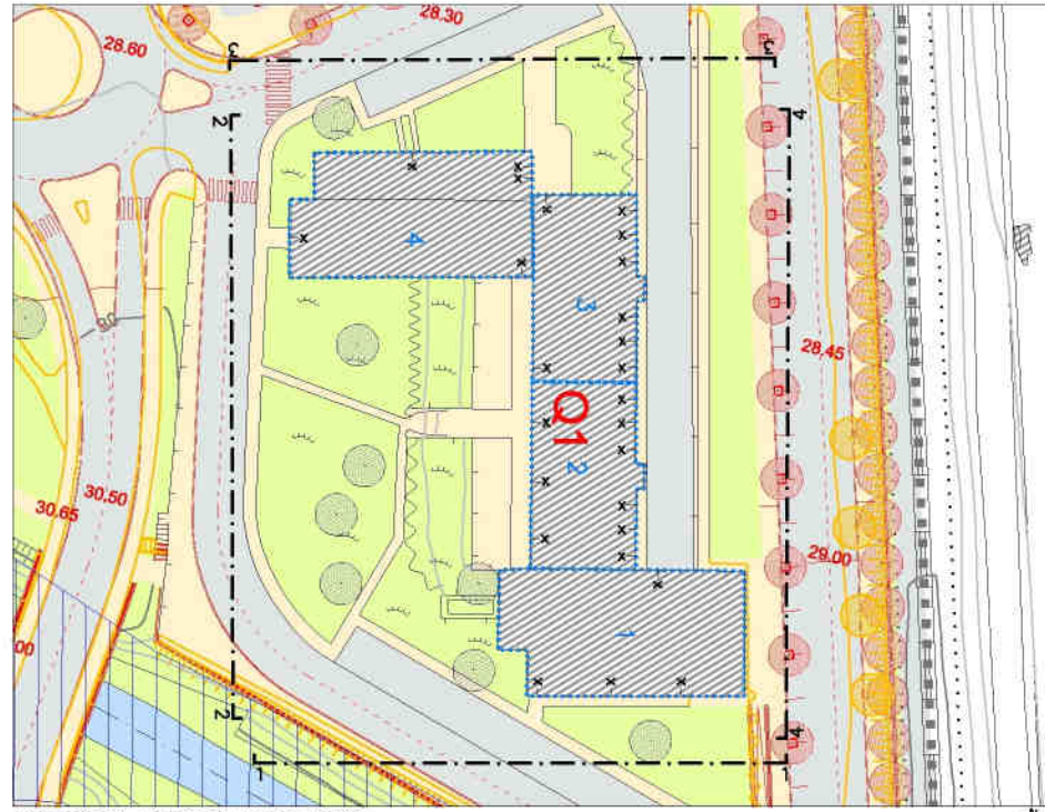
Extracto da Planta de Implantação
